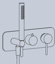
F3049WX2 Miscelatore incasso doccia a 2 uscite con set doccia Built-in shower mixer with 2 outlets and shower set
