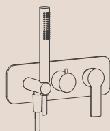
F3149WX2 Miscelatore incasso doccia a 2 uscite con set doccia Built-in shower mixer with 2 outlets and shower set
